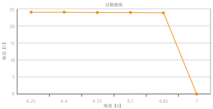
LM-150-24-G2D2
